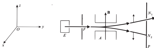
FIGURE 5 – Lorsque l'on perce un trou dans la plaque P à l'emplacement de la tache N_1 , les atomes qui passent par ce trou sont tous dans l'état de spin |+\rangle ; l'appareil de Stern et Gerlach fonctionne alors comme un polariseur.
