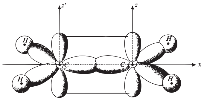
FIGURE 9 – Structure schématique de la molécule d'éthylène C_2H_4 . Les deux atomes de carbone forment entre eux une double liaison : une liaison \sigma assurée par des orbitales sp^2 du type de celles représentées sur la Figure 8 (les deux autres orbitales hybrides sp^2 à 120^\circ de la précédente assurant les liaisons C-H) ; une liaison \pi , due au recouvrement des orbitales p_z .
