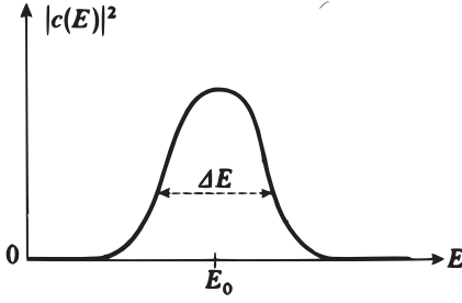
FIGURE 4 – En superposant des états stationnaires |\varphi_E\rangle avec des coefficients c(E) , on obtient un état |\psi\rangle du système où l'énergie n'est pas parfaitement définie ; l'incertitude \Delta E correspondante est donnée par la largeur de la courbe représentant |c(E)|^2 . D'après la quatrième relation d'incertitude (D-69), l'évolution de l'état |\psi(t)\rangle sera notable au bout d'un temps \Delta t tel que \Delta E \cdot \Delta t \gtrsim \hbar .
