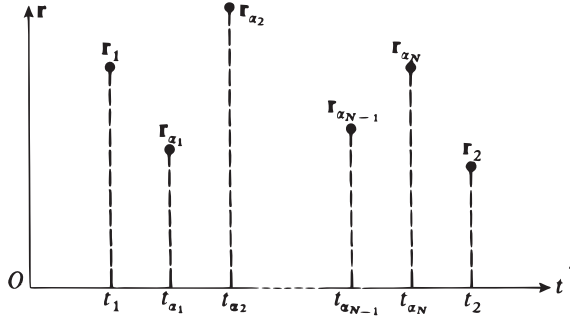
FIGURE 3 – Schéma associé à un “chemin d’espace-temps” : on prend N instants intermédiaires t_{\alpha_i} ( i = 1, 2, \dots, N ) régulièrement répartis entre t_1 , et t_2 , et on choisit pour chacun d’eux une valeur de \mathbf{r} .
