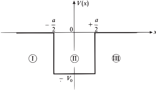
FIGURE 4 – Puits carré de potentiel.
