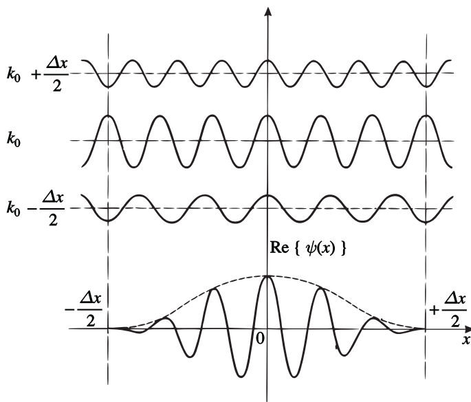
FIGURE 4 – Parties réelles des trois ondes dont la somme donne la fonction \psi(x) écrite en C-10. En x = 0 , les trois ondes sont en phase, de sorte qu'elles interfèrent constructivement ; lorsqu'on s'écarte de x = 0 , elles se déphasent les unes par rapport aux autres et interfèrent destructivement pour x = \pm \Delta x/2 . Sur la partie inférieure de la figure, on a représenté \text{Re}\{\psi(x)\} . La courbe en traits tiretés correspond à la fonction [1 + \cos(\frac{\Delta k}{2}x)] qui, d'après C-10, donne |\psi(x)| (c'est-à-dire la forme du paquet d'ondes).
