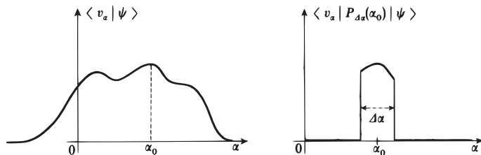
FIGURE 9 – Illustration du postulat de réduction du paquet d’ondes dans le cas d’un spectre continu : on mesure l’observable A , de vecteurs propres |v_a\rangle , et de valeurs propres \alpha . L’appareil de mesure a une sélectivité \Delta\alpha . Si la valeur trouvée est \alpha_0 , à \Delta\alpha près, l’effet de la mesure sur la fonction d’onde \langle v_a | \psi \rangle est de la “tronquer” autour de la valeur \alpha_0 (pour normer la nouvelle fonction d’onde, il faudrait évidemment la multiplier par un facteur plus grand que 1).
