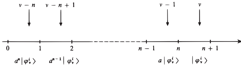
FIGURE 3 – En faisant agir l'opérateur a plusieurs fois sur le ket |\varphi_\nu^i\rangle , on construit des vecteurs propres de N de valeurs propres \nu - 1 , \nu - 2 , etc.
