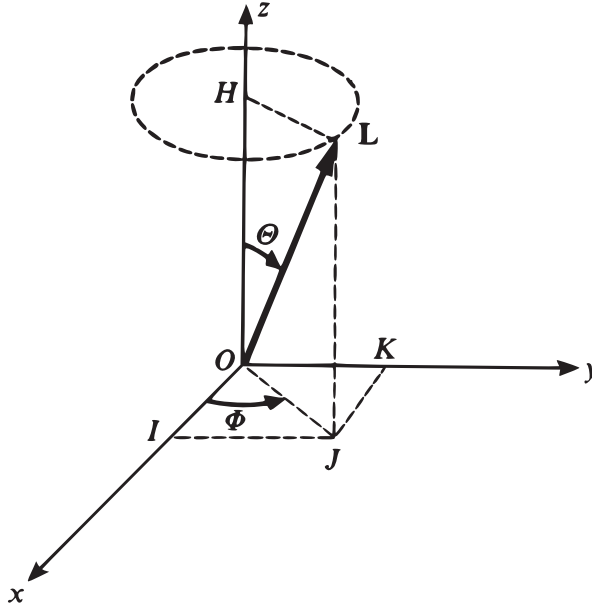
FIGURE 3 – Modèle classique pouvant être associé au moment cinétique orbital d'une particule dans un état |l, m\rangle . On suppose que la longueur |OL| et l'angle \Theta sont connus, mais que \Phi est une variable aléatoire dont la densité de probabilité est constante dans l'intervalle [0, 2\pi] ; les valeurs moyennes classiques des composantes de OL , ainsi que celles des carrés de ces composantes, sont alors égales aux valeurs moyennes quantiques correspondantes.
