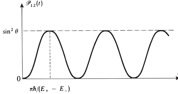
FIGURE 14 – Variations en fonction du temps de la probabilité \mathcal{P}_{12}(t) de trouver le système dans l'état |\varphi_2\rangle alors qu'il était initialement dans l'état |\varphi_1\rangle . Lorsque les états |\varphi_1\rangle et |\varphi_2\rangle ont même énergie non perturbée, la probabilité \mathcal{P}_{12}(t) peut atteindre la valeur 1.
