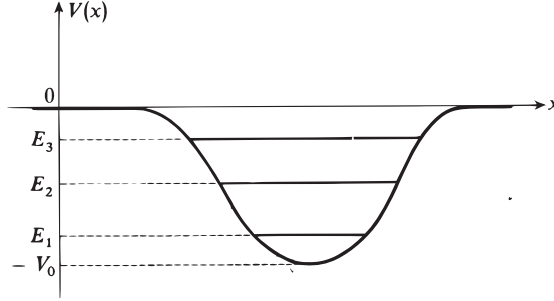
FIGURE 3 – Représentation schématisée des états liés d'une particule dans un puits de potentiel. Pour chacun de ces états stationnaires, on trace un trait horizontal dont l'ordonnée est égale à l'énergie du niveau correspondant. On limite ce trait aux points d'intersection avec la courbe représentant le potentiel V(x) , c'est-à-dire à la région où s'effectuerait le mouvement classique de même énergie ; ceci donne une idée de l'extension de la fonction d'onde.
