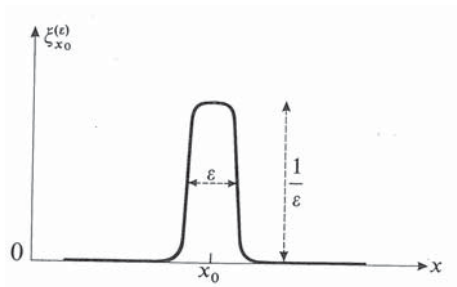
FIGURE 1 - \xi_{x_0}^{(\varepsilon)} est une fonction présentant un pic en x = x_0 (de largeur \varepsilon et de hauteur 1/\varepsilon ) et dont l'intégrale entre -\infty et +\infty est égale à l'unité.
