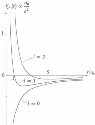
FIGURE 2 - Allure du potentiel effectif V_{\text{eff}}(r) pour les premières valeurs de l dans le cas où V(r) = -e^2/r . Lorsque l = 0 , V_{\text{eff}}(r) est simplement égal à V(r) ; lorsque l prend les valeurs 1, 2, etc., V_{\text{eff}}(r) est obtenu en ajoutant à V(r) le potentiel centrifuge l(l+1)\hbar^2/2\mu r^2 , qui tend vers +\infty lorsque r tend vers zéro.
