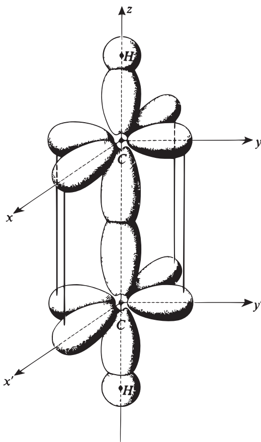
FIGURE 7 – Structure schématique de la molécule d’acétylène C_2H_2 . Pour chaque atome de carbone, deux électrons se trouvent dans les orbitales hybrides sp_z (cf. Fig. 6), et contribuent aux liaisons C-H et C-C (liaison \sigma ) ; de plus, deux électrons sont dans des orbitales p_x et p_y , et assurent des liaisons supplémentaires entre les deux atomes de carbone (liaisons \pi , plus faibles que les liaisons \sigma ), schématisées par des barres verticales sur la figure. La liaison C-C est donc une “triple liaison”.
