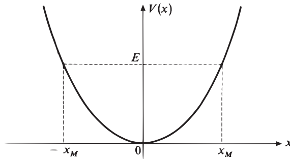
FIGURE 1 – Énergie potentielle V(x) d'un oscillateur harmonique à une dimension. L'amplitude d'un mouvement classique d'énergie E est x_M .
