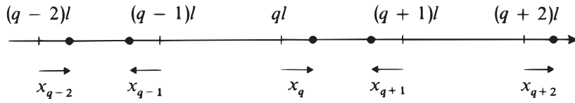
FIGURE 4 – Les modes k = \pm\pi/l sont ceux où deux oscillateurs voisins se déplacent en opposition de phase; le couplage V modifie alors fortement leur fréquence.
