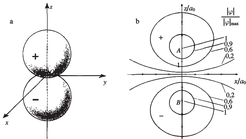
FIGURE 2 – Deux représentations possibles d'une orbitale p_z ( l = 1, m = 0 ) fig. a : dépendance angulaire de cette orbitale : dans chaque direction \theta, \varphi , on porte |\varphi_{n,l=1,m=0}(r, \theta, \varphi)| , r étant fixé. On obtient ainsi deux sphères tangentes en O au plan xOy , le signe indiqué sur chacune d'elles étant celui de la fonction d'onde (qui est réelle).
