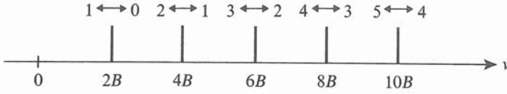
FIGURE 3 – Fréquences apparaissant dans l'évolution de la valeur moyenne de l'observable Z . Du fait de la règle de sélection \Delta l = \pm 1 , seules interviennent les fréquences de Bohr 2Bl (avec l \geq 1 ) associées à deux niveaux E_l et E_{l-1} adjacents sur la Figure 2.
