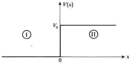
FIGURE 1 – Marche de potentiel de hauteur V_0 .
