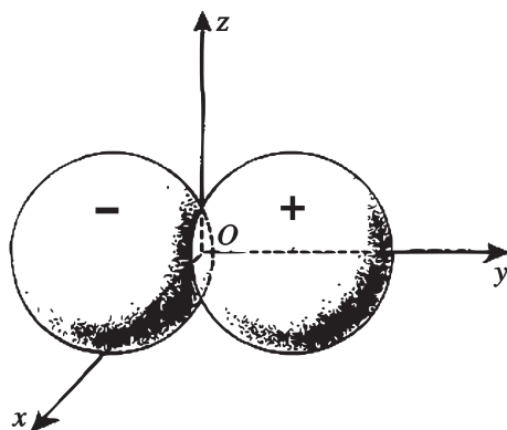
FIGURE 4 – Dépendance angulaire d'une orbitale p_y .
