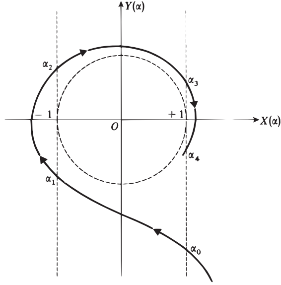
FIGURE 2 – Variations en fonction de \alpha du nombre complexe e^{i\alpha l}F(\alpha) = X(\alpha) + iY(\alpha) . Comme |F(\alpha)| > 1 , la courbe obtenue dans le plan complexe est extérieure au cercle de centre O et de rayon unité. La discussion qui suit montre que si |X(\alpha)| est inférieur à 1, c'est-à-dire si la valeur de \alpha choisie donne un point de la courbe compris entre les deux droites verticales en traits tiretés de la figure, l'énergie correspondante tombe dans une "bande permise"; dans le cas contraire, elle tombe dans une "bande interdite".
