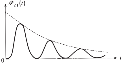
FIGURE 1 – Effet d'un couplage fort entre un état stable |\varphi_2\rangle et un état instable |\varphi_1\rangle : si le système est initialement dans l'état |\varphi_2\rangle , la probabilité \mathcal{P}_{21}(t) de le trouver à l'instant t dans l'état |\varphi_1\rangle présente des oscillations amorties.
