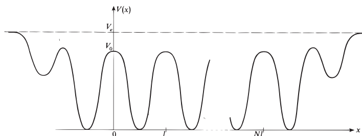
FIGURE 3 – Variations en fonction de x du potentiel vu par un électron dans un "cristal à une dimension" et sur ses bords. À l'intérieur du cristal, le potentiel a une structure périodique; V(x) est maximal entre les ions (barrières en x = 0, l, 2l, \dots ), minimal aux positions des ions (puits en x = l/2, 3l/2, \dots ). Sur les bords du cristal, V(x) varie de manière plus ou moins compliquée sur une distance comparable à l , puis tend rapidement vers une valeur constante V_e .
