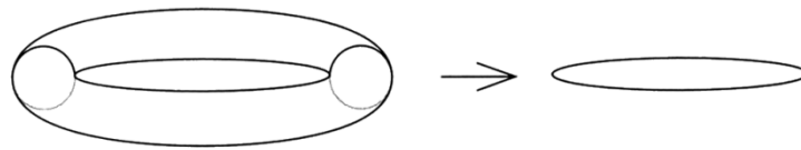
Figure 10. Sur la gauche, nous avons une membrane bidimensionnelle, que nous pouvons imaginer être enroulée autour d’une dimension cachée, ici un petit cercle. Vu de suffisamment loin (à gauche), cela ressemble à une corde enroulée autour de la dimension plus grande.
