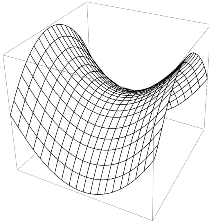
Figure 12. Une surface en « selle de cheval », ce qui correspond à la géométrie de l'espace dans un univers où l'énergie noire est négative.
