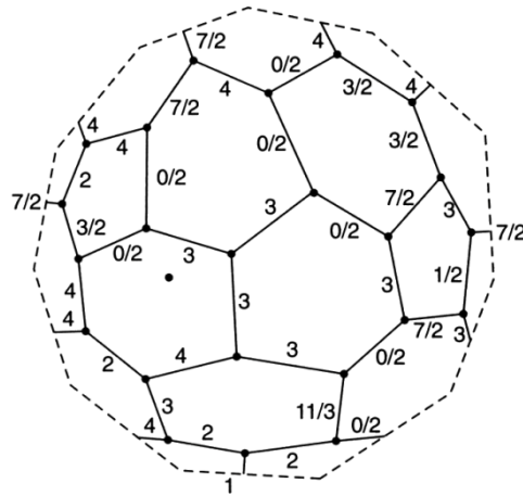
Figures 15. Un réseau de spin, qui est l'état de la géométrie quantique dans la gravité quantique à boucles et les théories qui lui sont liées. Des quanta de volume sont associés aux nœuds et des quantas de surface sont associés aux arêtes.
