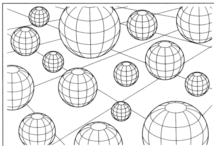
Figure 8. La géométrie des dimensions cachées peut varier dans l'espace et le temps. Ici, le rayon des sphères varie.
