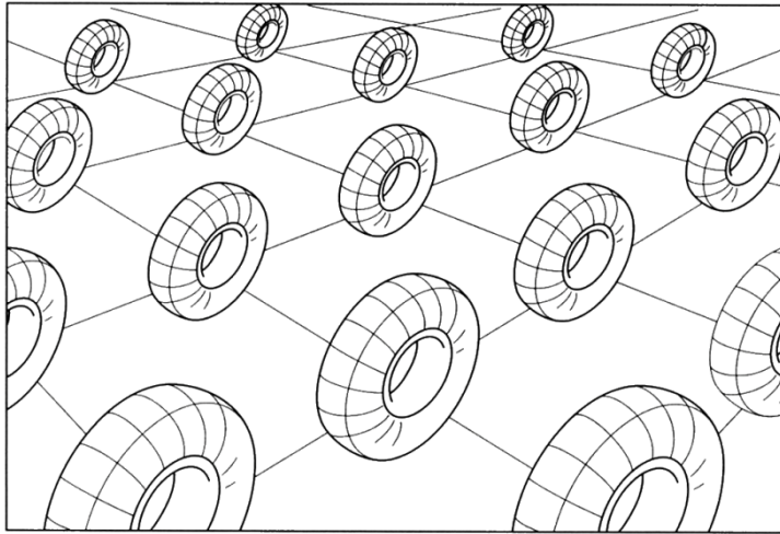
Figure 7. Les dimensions cachées admettent différentes topologies. Ici, deux dimensions cachées adoptent la forme d'un beignet, ou tore .
