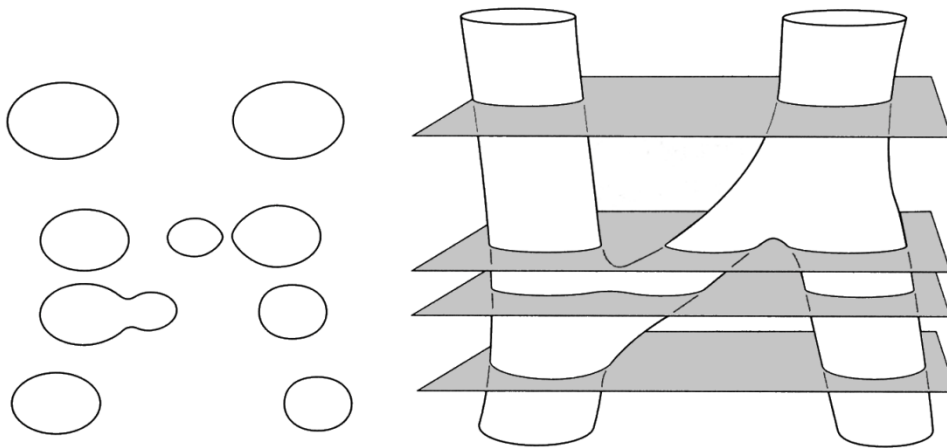
Figure 6. La propagation et l'interaction des cordes sont déterminées par la même loi, qui stipule que l'aire de la surface spatio-temporelle dessinée par les cordes doit être minimale.
