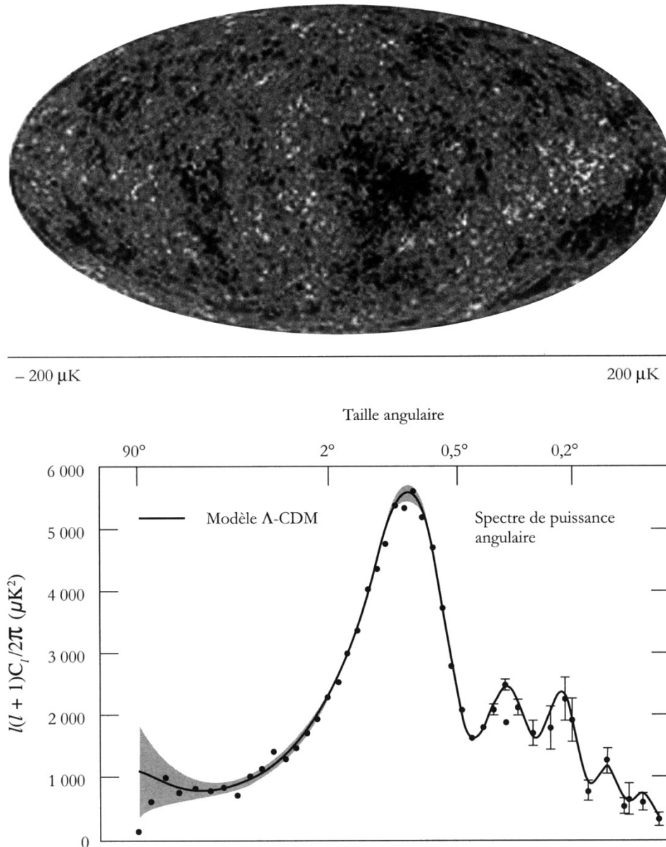
Figure 13. En haut : le ciel vu aux fréquences micro-ondes. Le signal correspondant à notre galaxie a été supprimé, laissant une image de l'Univers tel qu'il était lorsqu'il fut suffisamment froid pour permettre aux protons et aux électrons de se rassembler et ainsi créer de l'hydrogène. En bas : la distribution de l'énergie de l'image du haut à différentes longueurs d'ondes. Les points représentent les données du WMAP et d'autres observations. La courbe représente les prédictions du modèle standard cosmologique.
