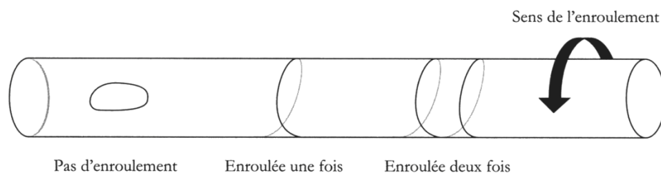
Figure 9. Les cordes peuvent s'enrouler autour d'une dimension cachée.
