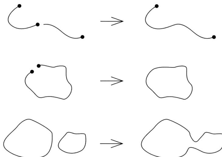
Figures 5. En haut : deux cordes ouvertes joignent une de leur extrémité. Au milieu : les deux extrémités d'une corde ouverte se joignent pour former une corde fermée. En bas : deux cordes fermées se joignent pour former une seule corde fermée.
