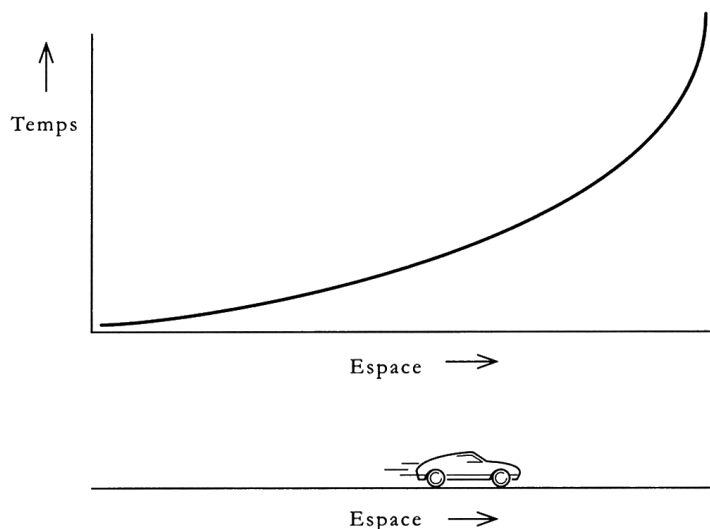
Figure 3. Une voiture décélérant sur une ligne droite de l'espace parcourt une courbe dans l'espace-temps.
