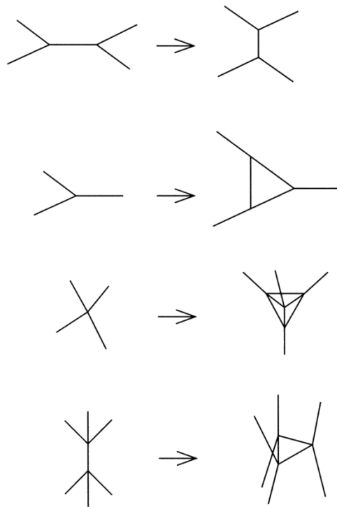
Figure 16. Les réseaux de spin évoluent dans le temps selon une série de changements locaux tels que ceux représentés ici.
