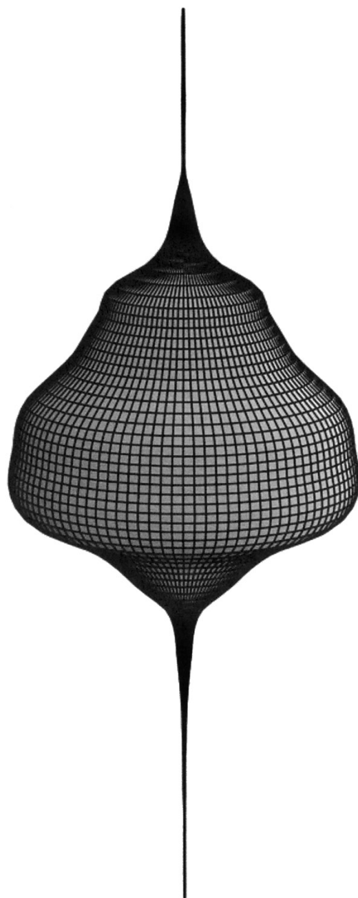
Figure 14. Un modèle d'univers quantique selon la triangulation dynamique causale.
