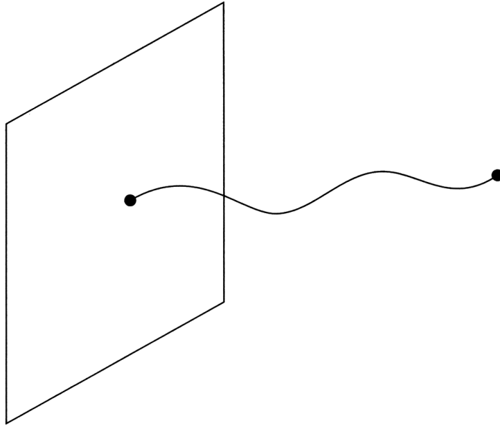
Figure 11. Une brane bidimensionnelle, sur laquelle une corde ouverte se termine.
