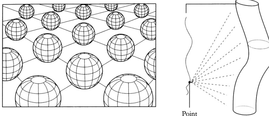
Figures 4. Les dimensions supplémentaires courbées de la théorie de Kaluza-Klein.
