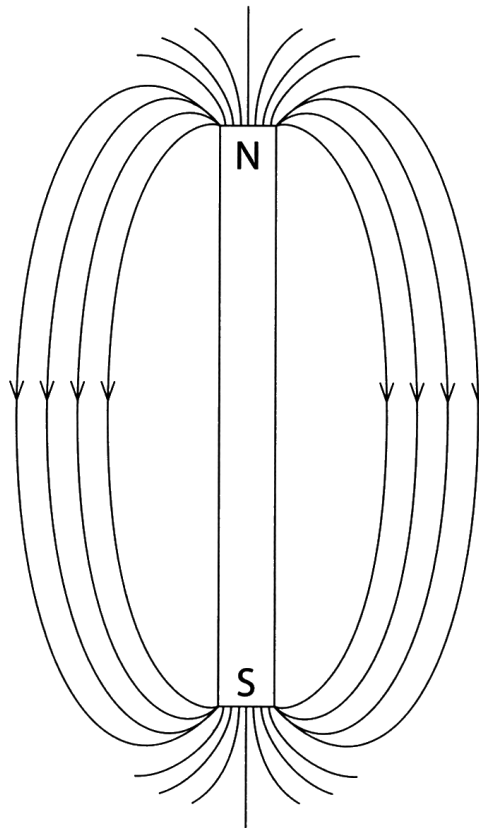
Figure 2. Des lignes de force dessinent le champ magnétique issu d'un aimant.
